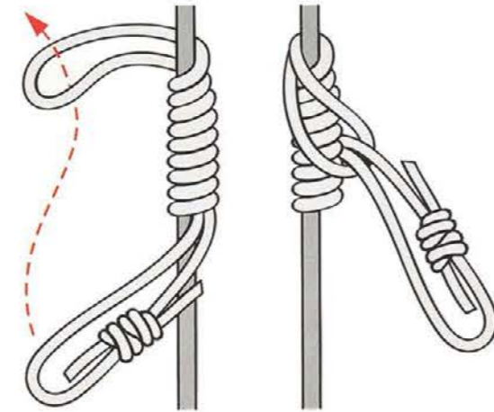
ASYMMETRICAL(MACHARD/FRENCH) PRUSIK KNOT
